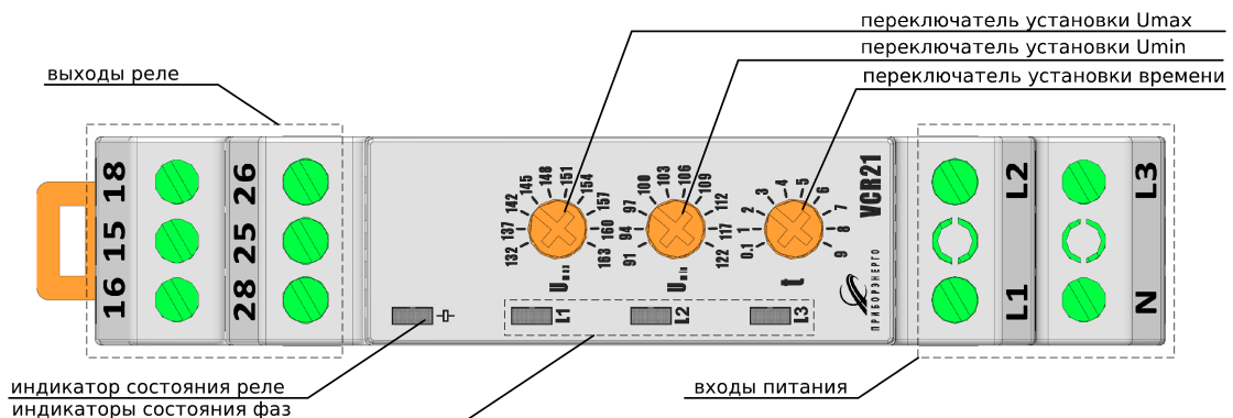
Рис.2 Панель управления и индикации реле контроля напряжения VCR21
