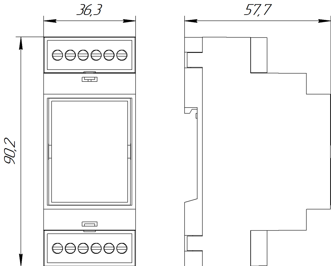
Рис. 3. Габаритные размеры Блока Инжекции.
